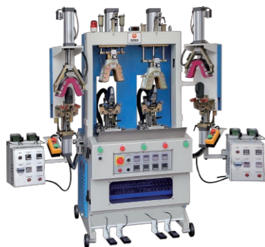
MT-518-2CQZ2HZ4A Máy Tạo Hình Gót Bốn Đầu Kích Hoạt Hai Nóng Hai Lạnh Two Cold Two Hot With Four Activation Heel Moulding Machine
